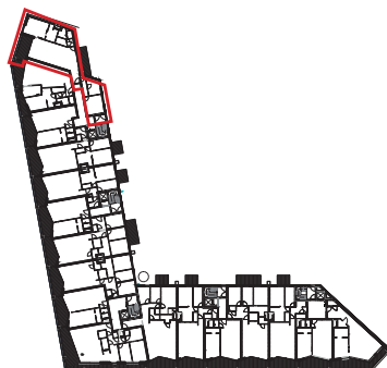
verdieping 1
